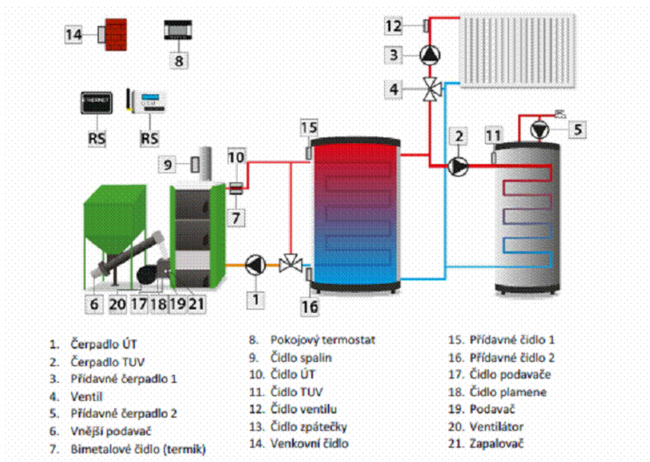
Zapojení kotle (přestavbové sady) s akumulací
